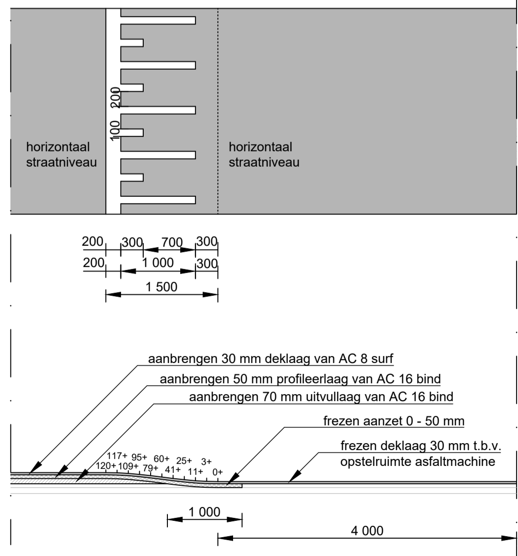
Verkeersplateau in asfalt 30 km/h; 120 mm hoog schaal 1:50
