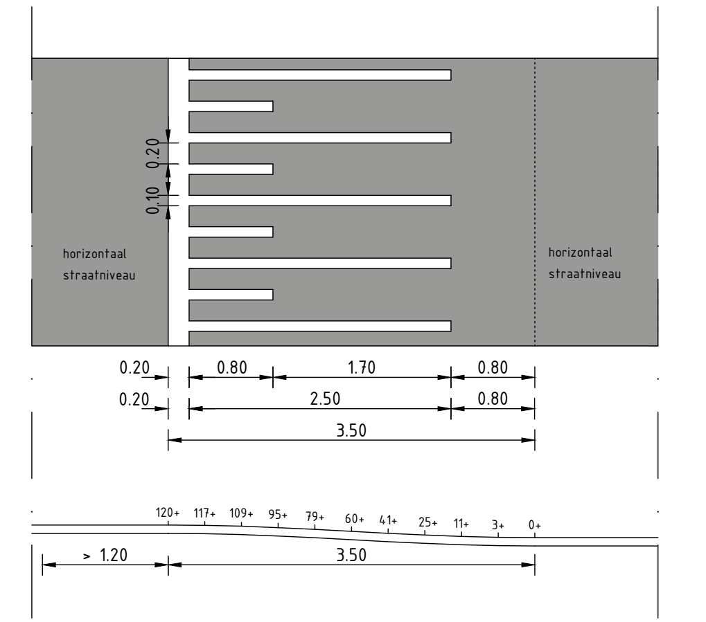
Verkeersplateau asfalt markering 50 km/h; 120 mm hoog Schaal 1:50
