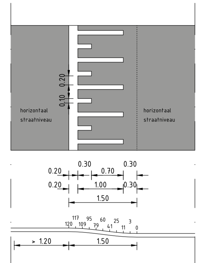
Verkeersplateau asfalt markering 30 km/h; 120 mm hoog Schaal 150
