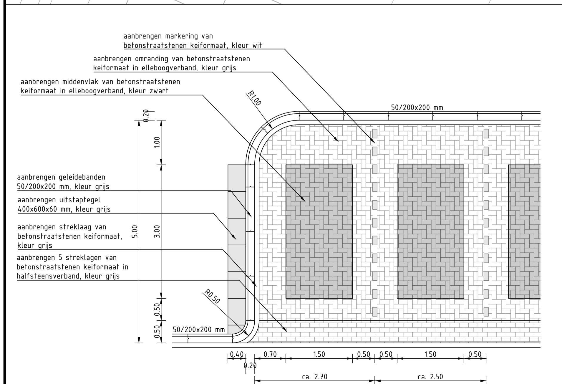
Principe-detail haaksparkeren schaal 1:50
